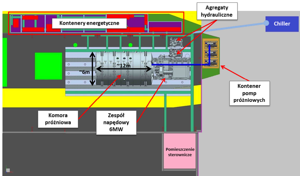
Rysunek 1 Plan rozmieszczenia komponentów laboratorium badawczego - rzut z góry.
