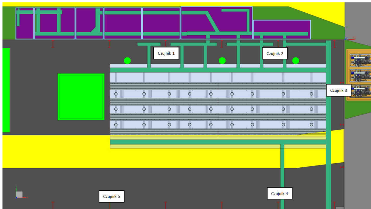
Rysunek 34 Rozmieszczenie urządzeń do pomiaru parametrów otoczenia na Hali Testów.
