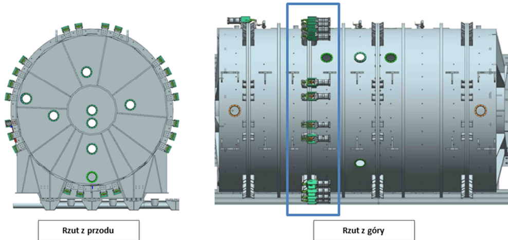
Rysunek 14 Rozmieszczenie siłowników domykających na komorze próżniowej.
