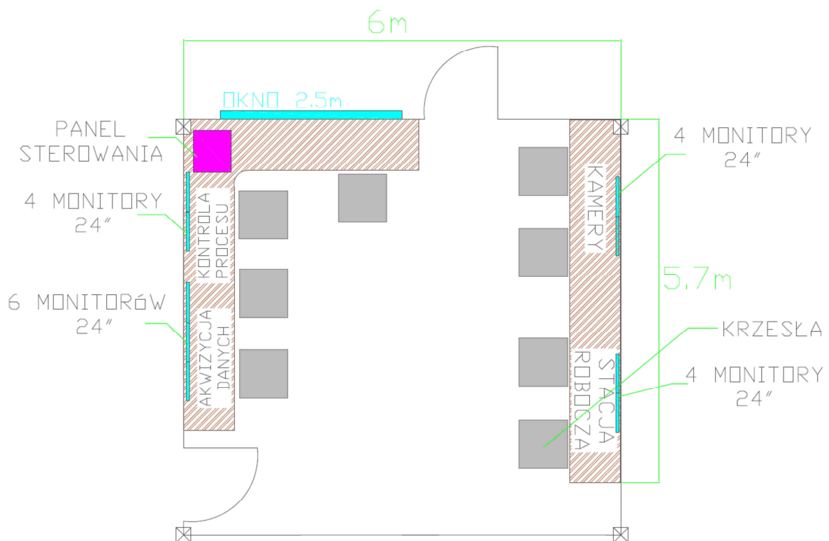
Rysunek 32 Rzut pomieszczenia sterowania wraz z planowaną zabudową meblową.
