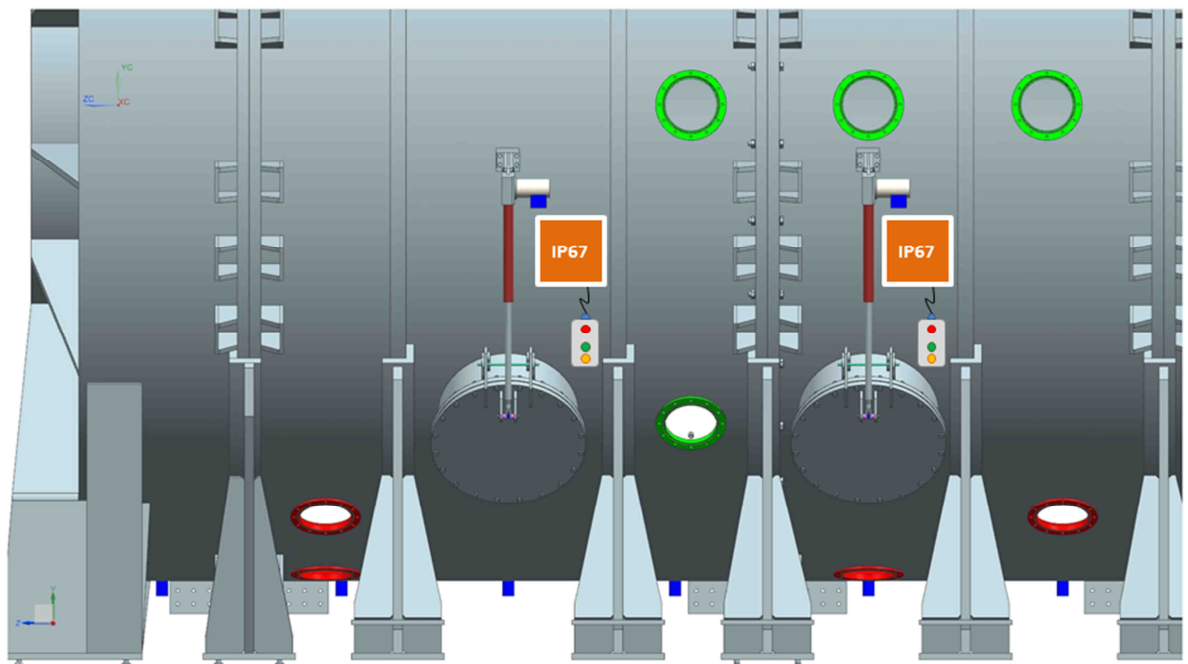
Rysunek 25 Planowane umieszczenie lokalnych skrzynek sterowania siłownikami włączów serwisowych.
